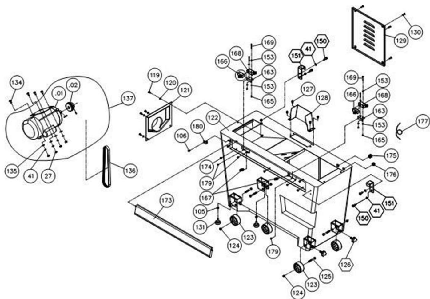
Чертеж №3 Корпус и двигатель
