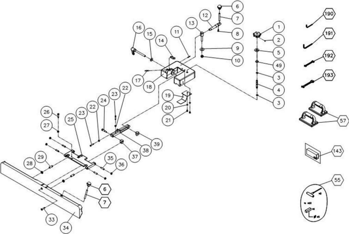
Чертеж №2 Параллельный упор
